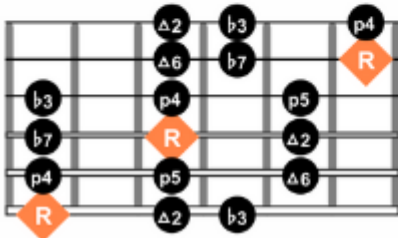
Phrygian mode
